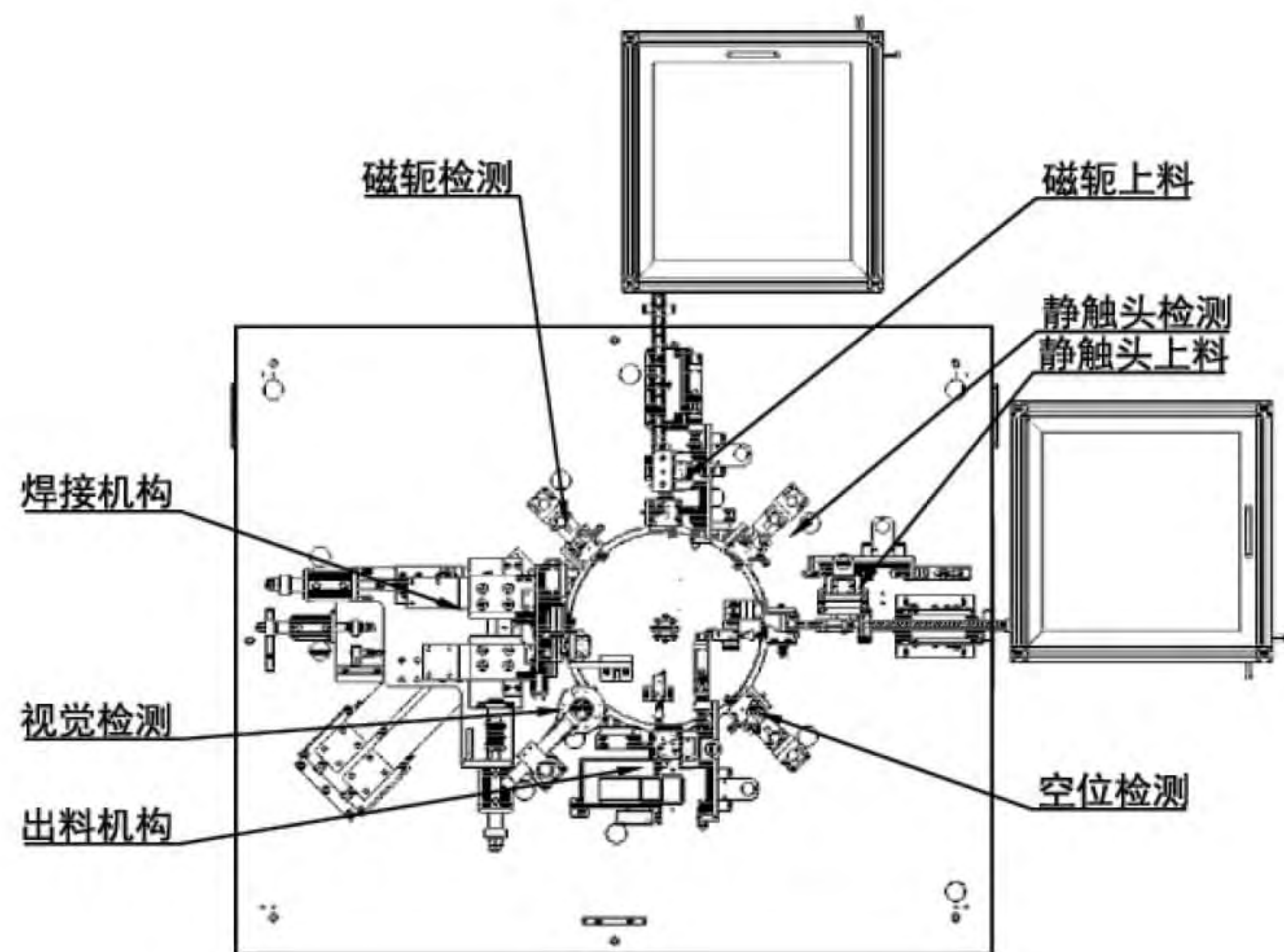
◎ 平面布置图 /layout plan
