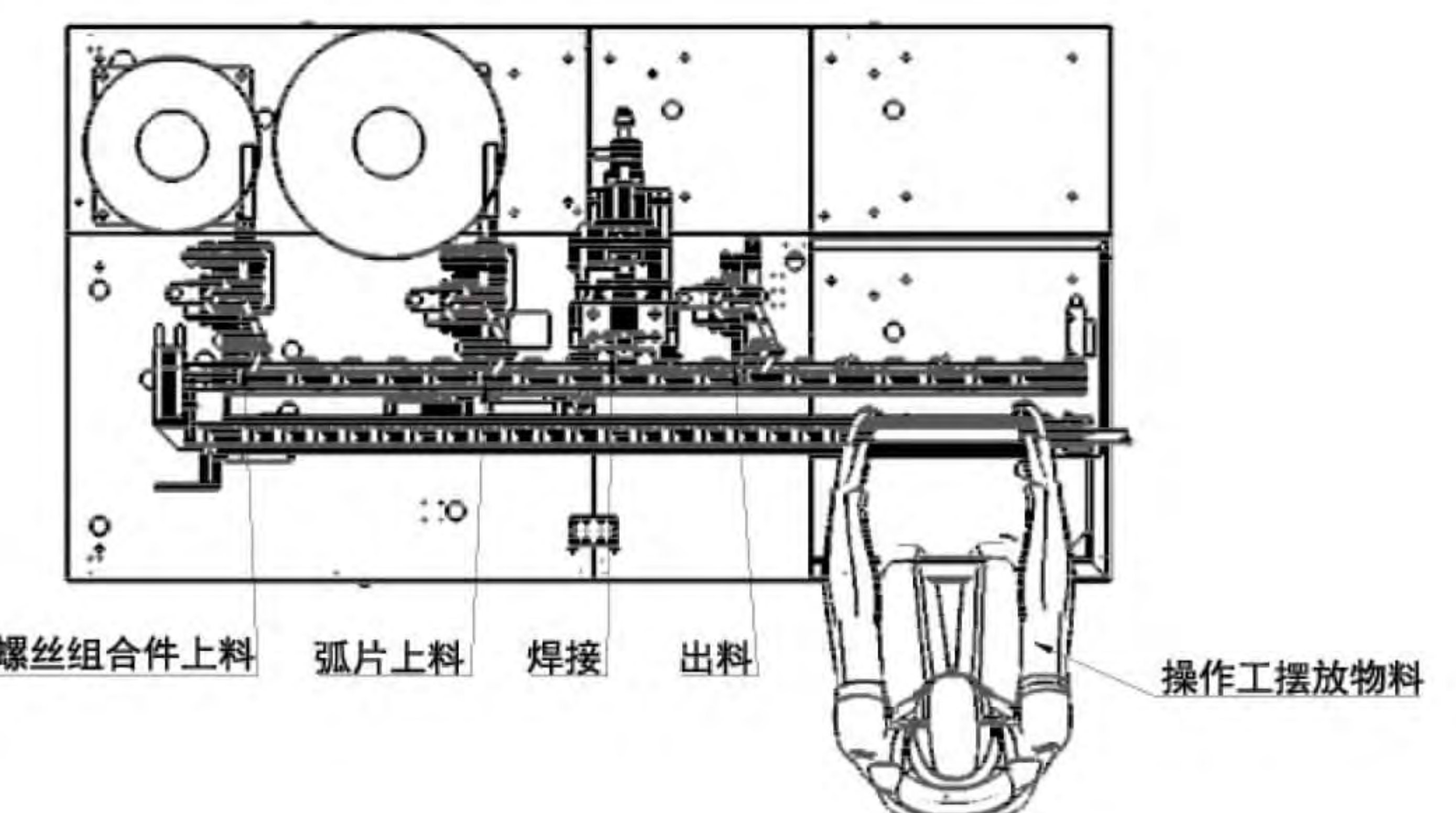
◎ 平面布置图 /layout plan
