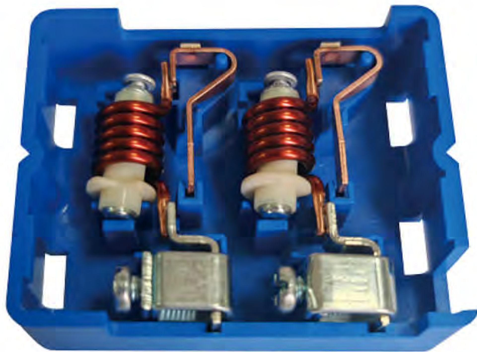
部分产品展示 /Some full products
