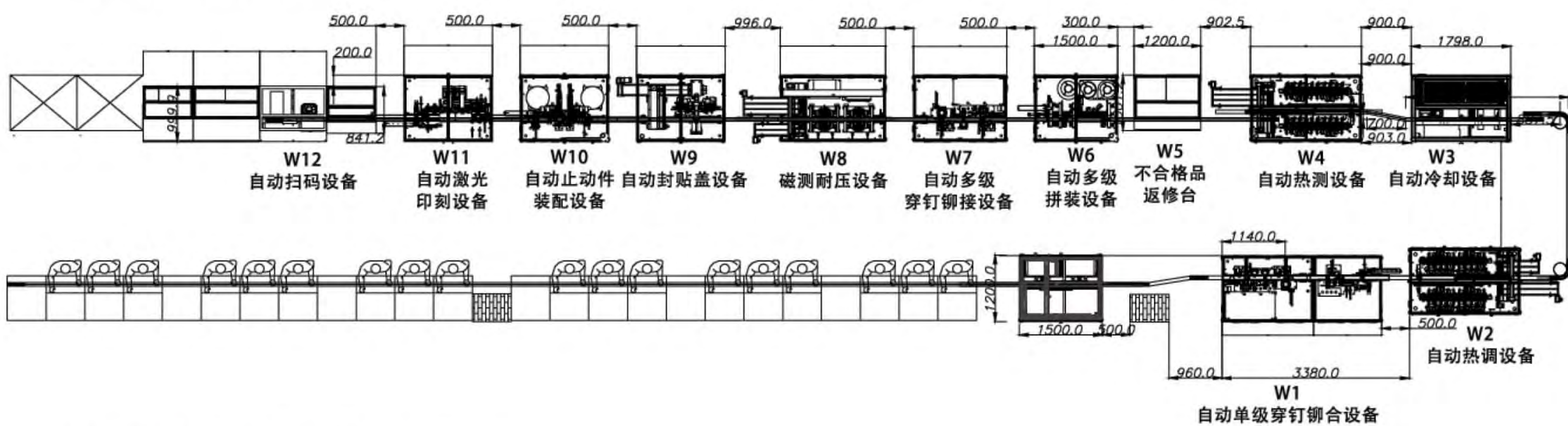
◎ 平面布置图 / layout plan
