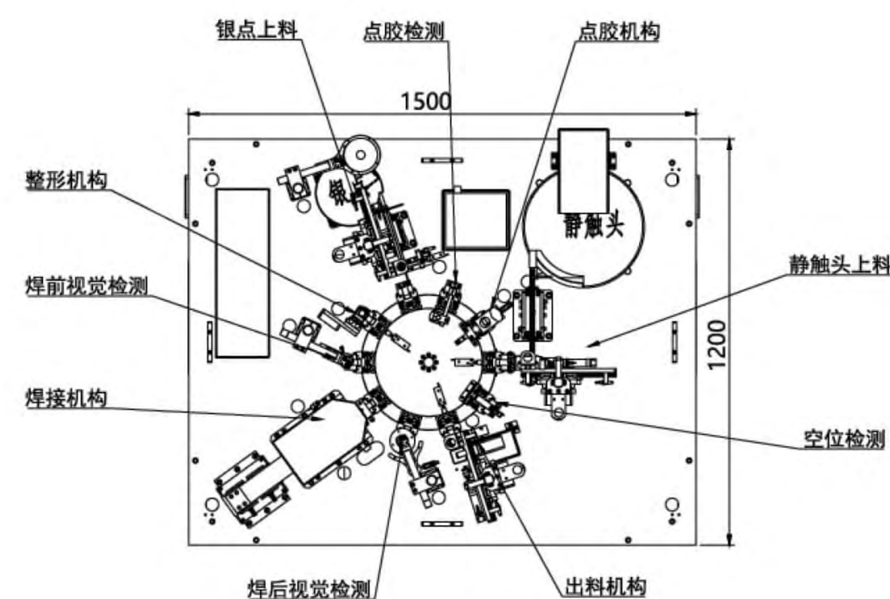
◎ 平面布置图 /layout plan
