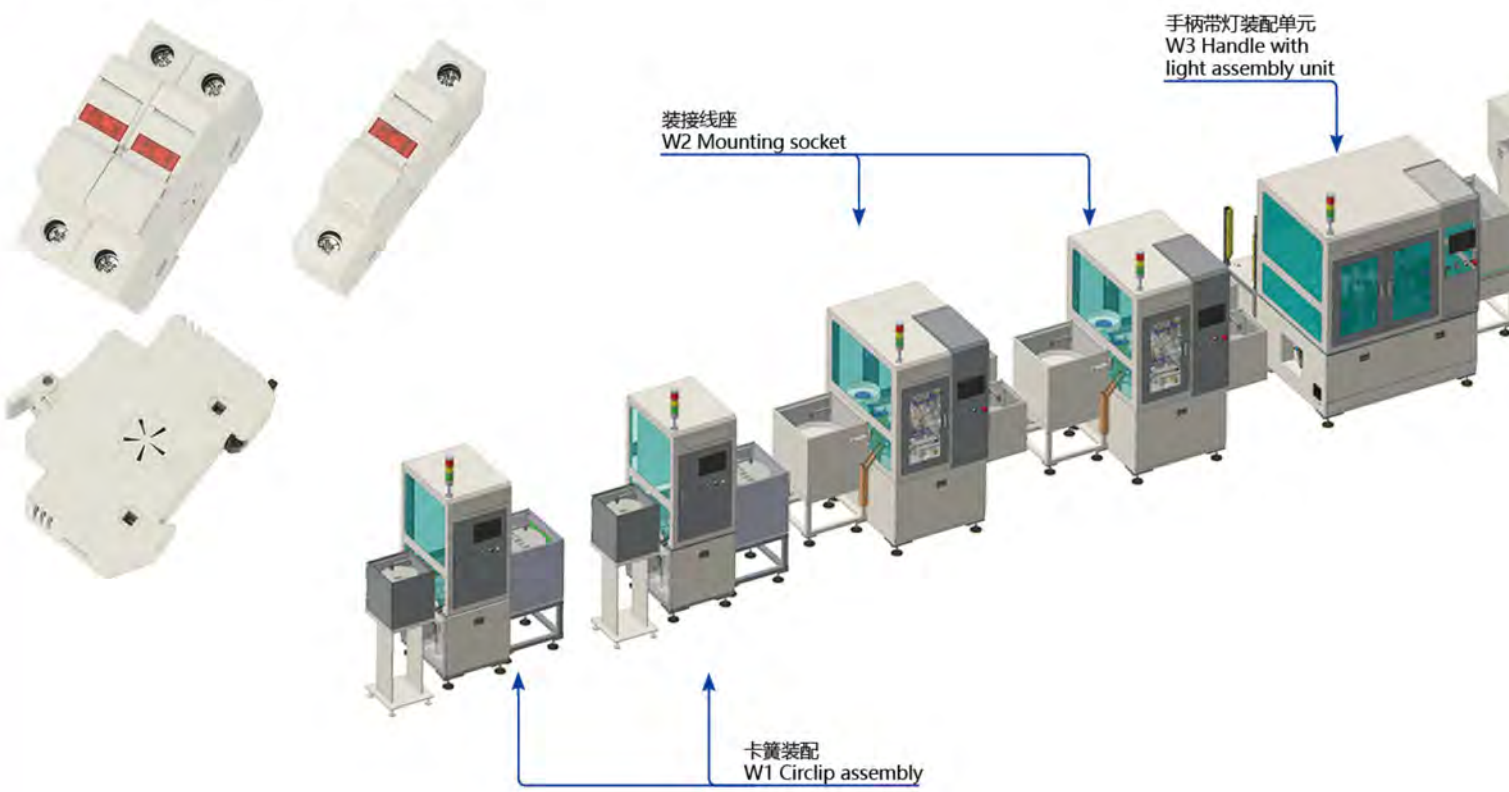
◎ 部分产品展示 /Some full products
