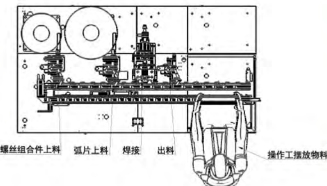
◎ 平面布置图 /layout plan
