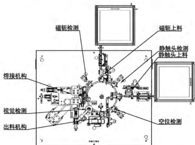
◎ 平面布置图 / layout plan
