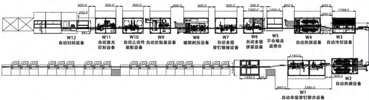
◎ 平面布置图 / layout plan
