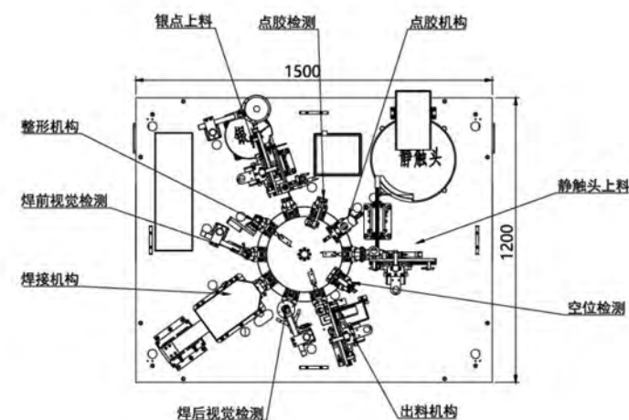
◎ 平面布置图 /layout plan
